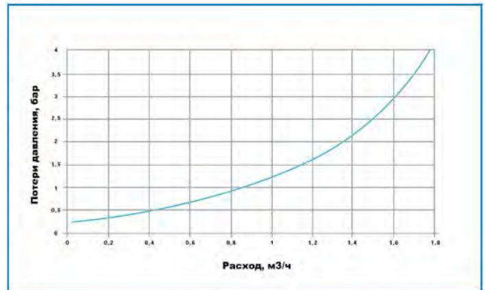
Диаграмма расход / потери давления
