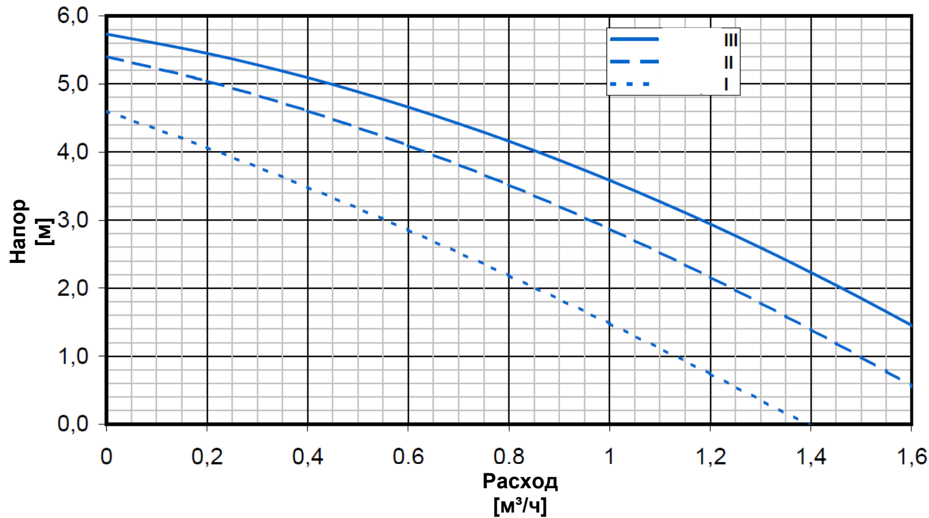
WILO RS 15/4-3
