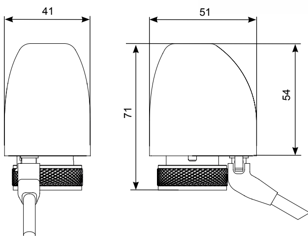
Размеры (мм)
