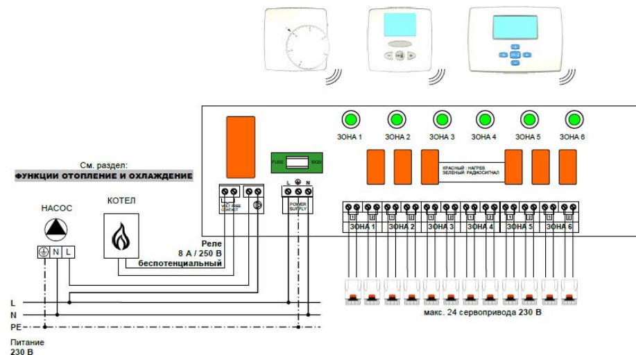
Схема подключения модуля на 6 зон.
